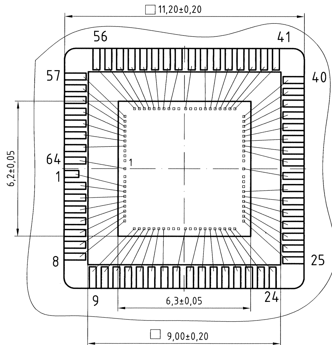
Б (10:1) Крышка и внешние выводы микросхемы не показаны
