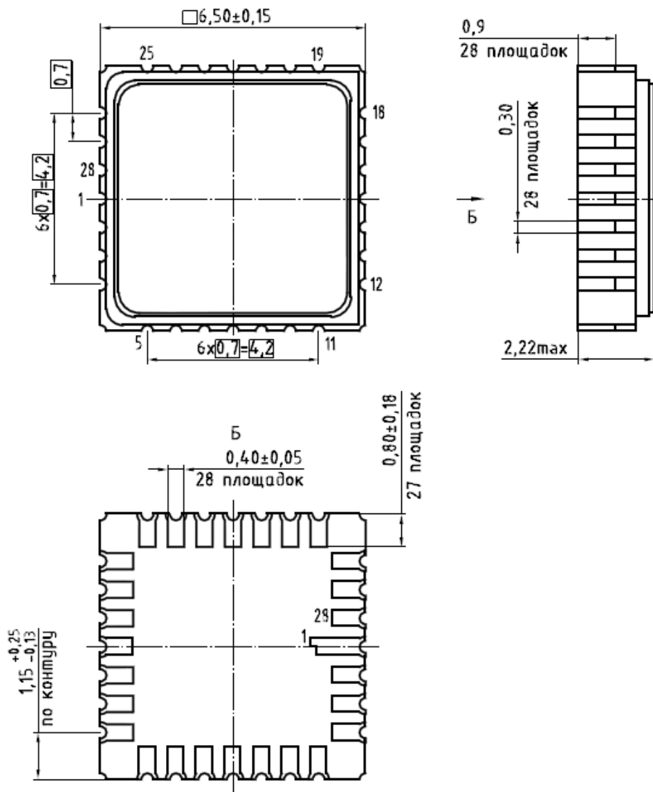
Рисунок 15.2 - Чертеж корпуса МК 5123.28-1.01
