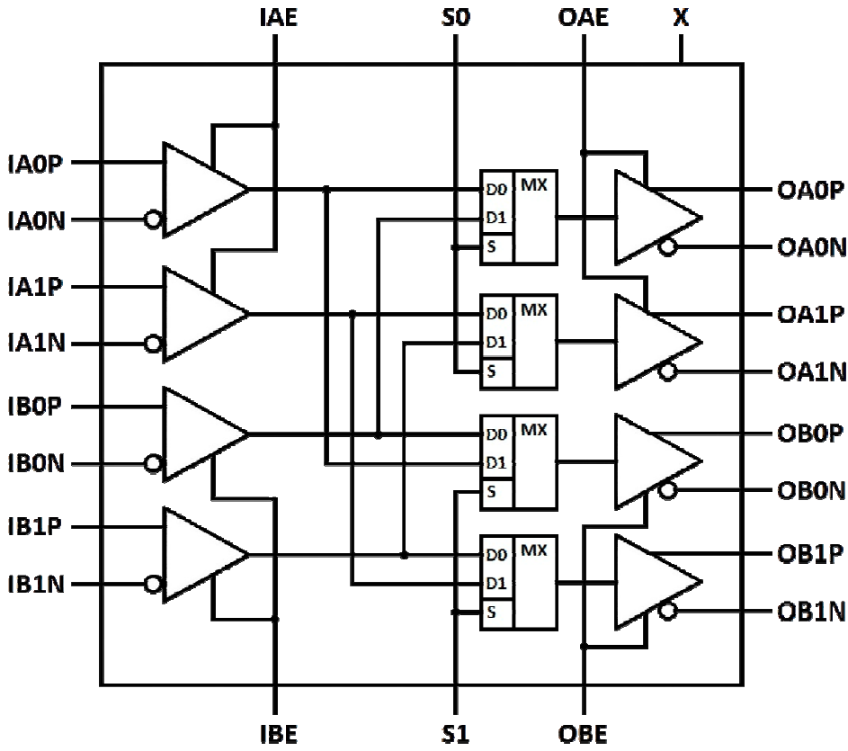
Рисунок 15.1 – Функциональная схема
